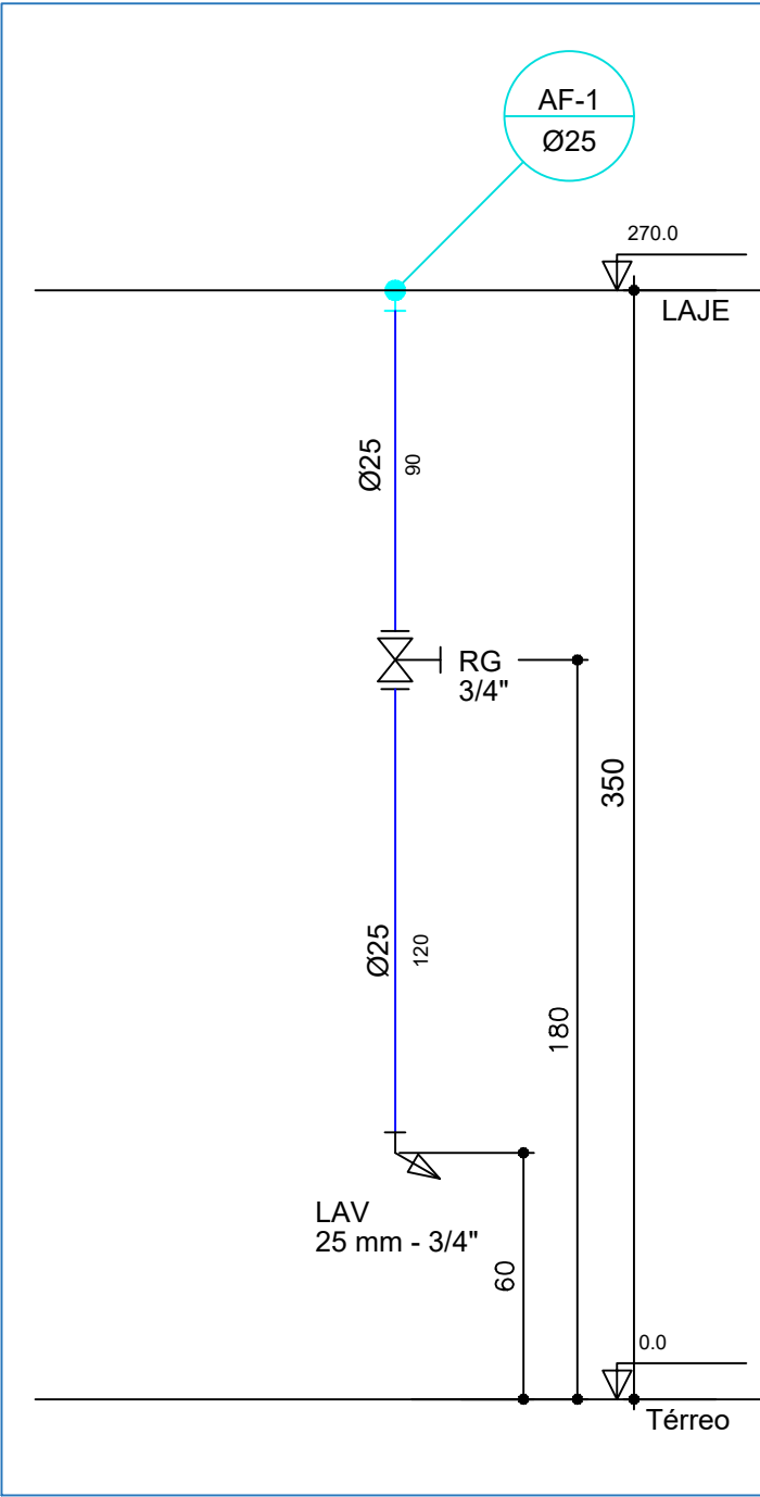
Wc Masc. escala 1:25
