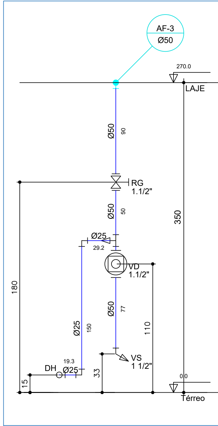
Wc Fem. escala 1:25
